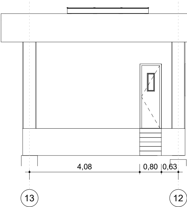
② T. SAMPING KIRI R. GENSET 1 : 80
