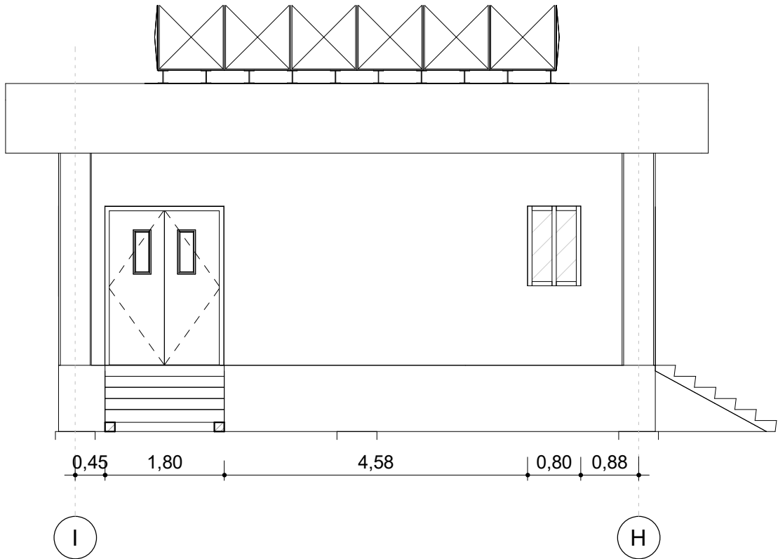
③ T. BELAKANG R. GENSET 1 : 80
