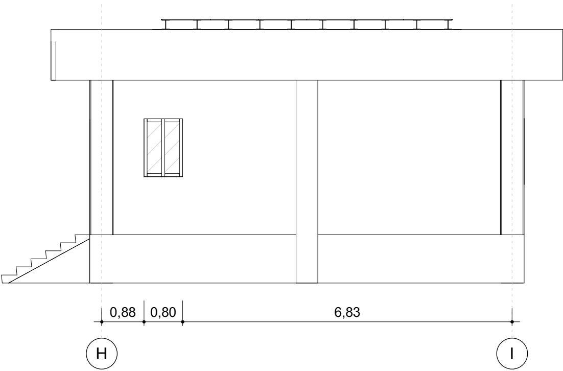
⑤ T. DEPAN R. GENSET 1 : 80
