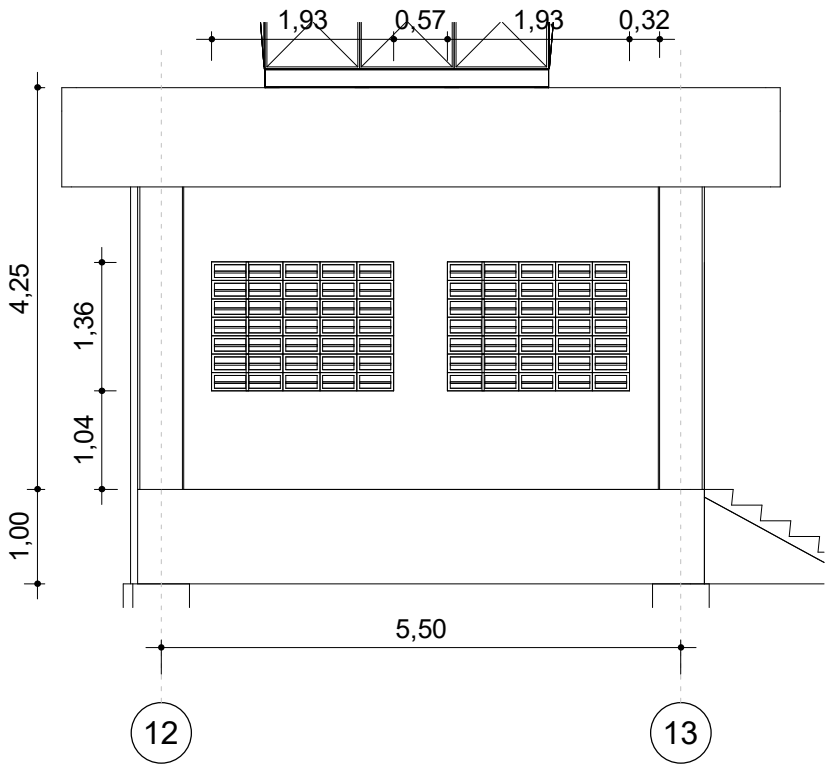
④ T. SAMPING KANAN R. GENSET 1 : 80
