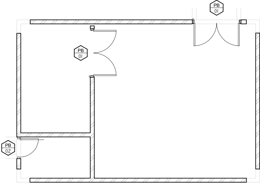
1 Pintu (R. Genset ) 1 : 80
